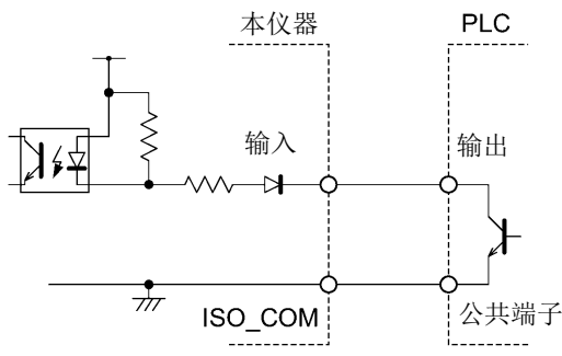
与 PLC 输出（负公共端子输出）的连接
