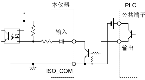
与 PLC 输出（正公共端子输出）的连接
