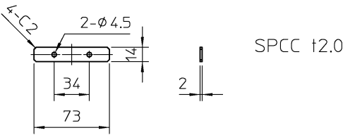
垫片（使用 2 片）
