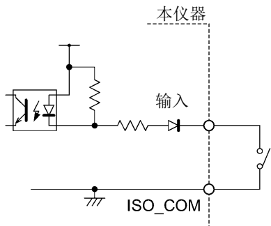
与开关的连接
