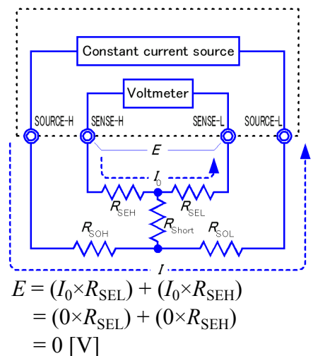
图 1 相近地连接 0\Omega 的状态
