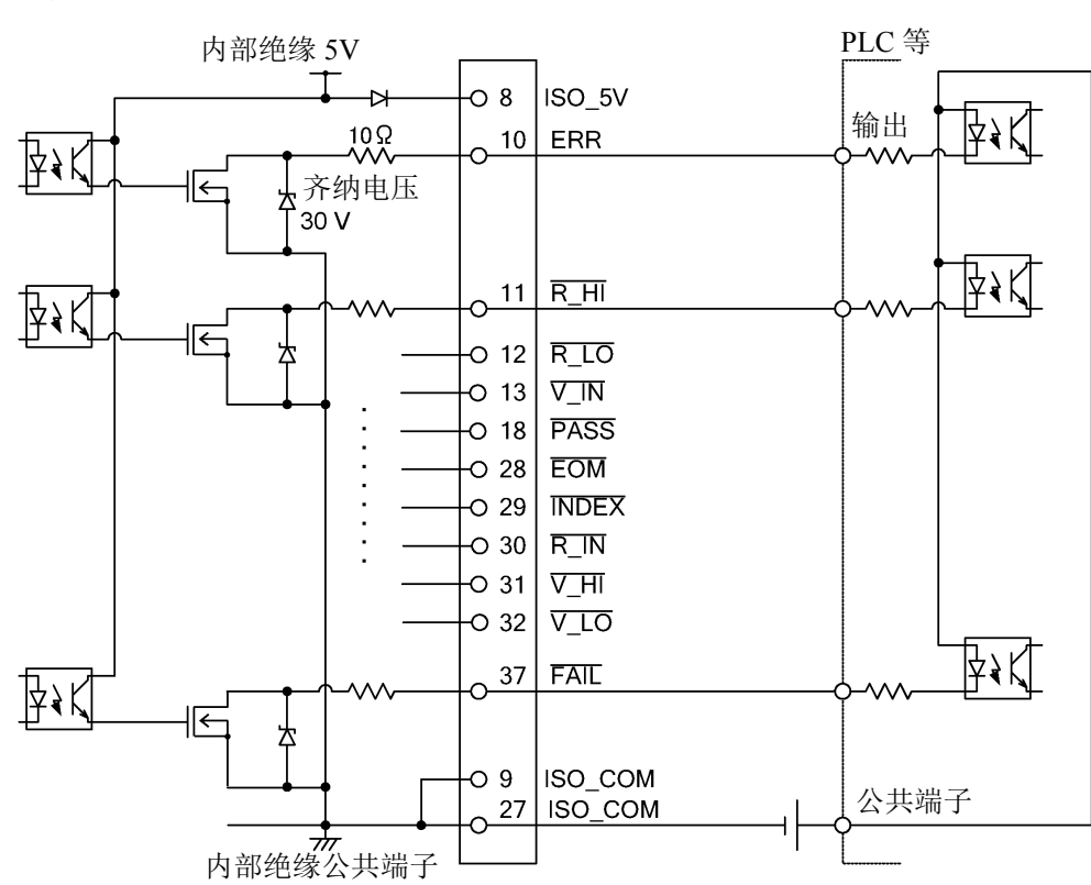
输出电路
